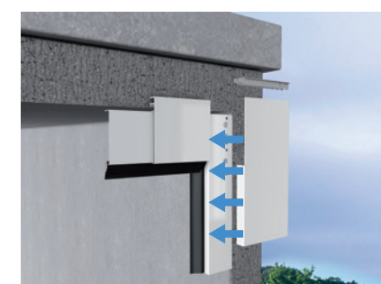
Universal-Blendenlösung, Außenansicht
