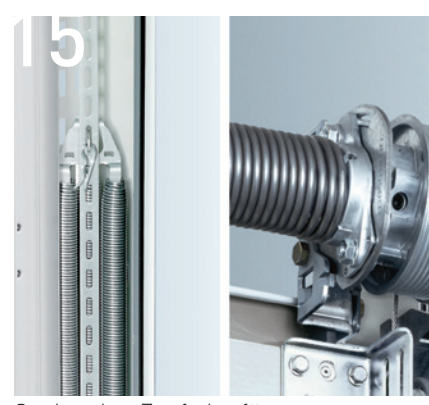
15 Senkrechte Zugfeder für Garagen-Sektionaltore
