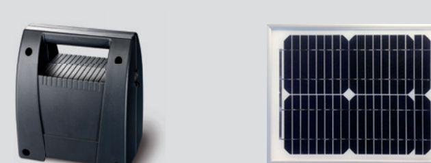
Akku-Pack Nennspannung 12 V DC, Nennkapazität 15 Ah, Nutzungsdauer 40 Tage bei max. 4 Öffnungen pro Tag und bei einer Temperatur von 20 °C, Temperaturbereich - 15 ° bis + 45 °C, integrierter Laderegler für Steckernetzteil • Geeignet für: Novomatic 423 Accu
